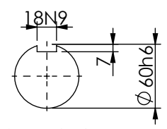
剖面 A-A
